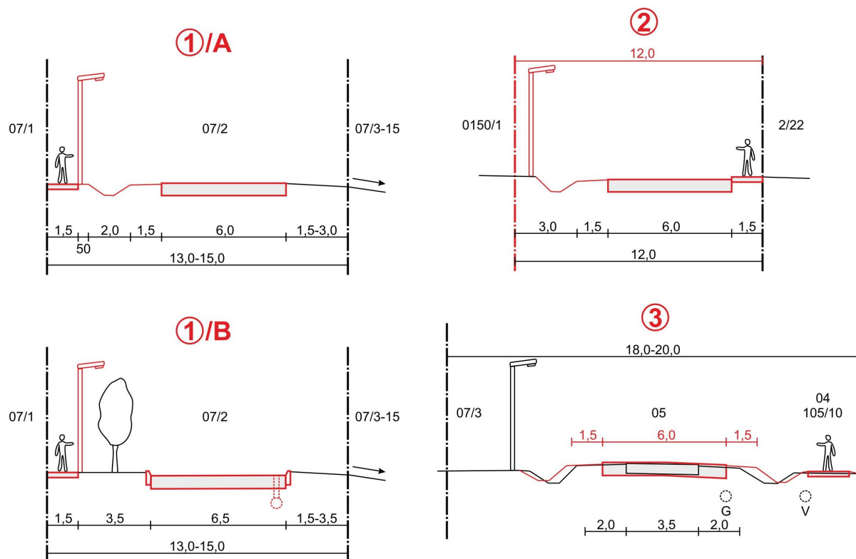
Az üdülőterület kiszolgáló útjának helyszínrajza és jellemző keresztmetsvényei
