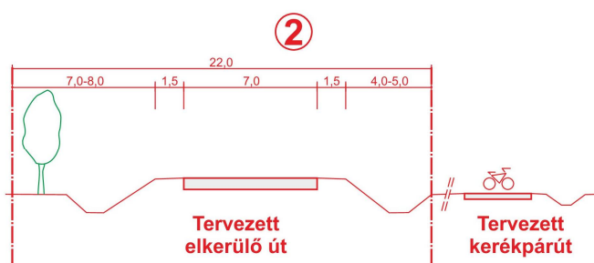
Jellemző keresztmetszvény a kerékpárút mellett
